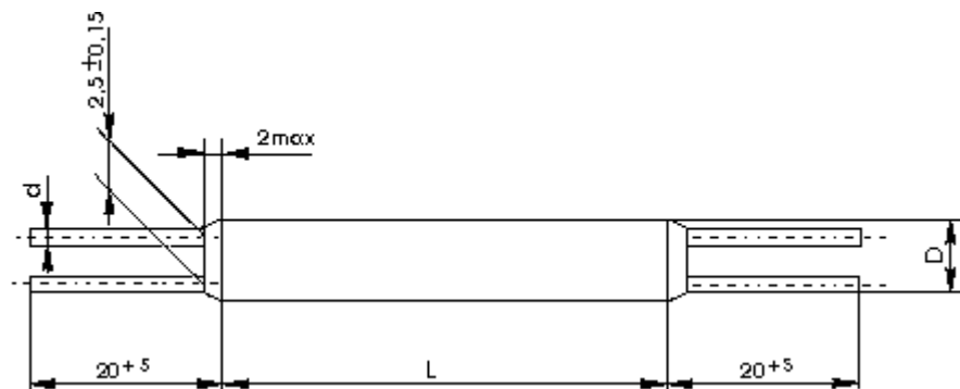
Резистор C5-42BВ:
