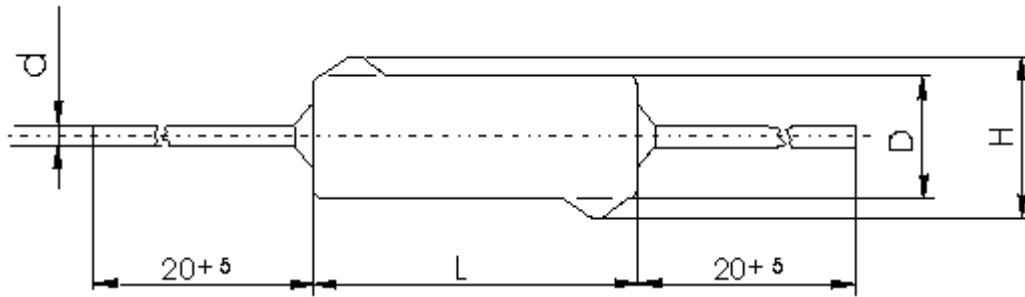
Резистор C5-42B:
